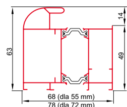
ościeznica aluminiowa z przekładką termiczną
