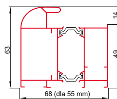
ościeżnica aluminiowa z przegrodą termiczną
