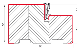
ościeznica stalowo-drewniana do drzwi 55 i 72 mm
