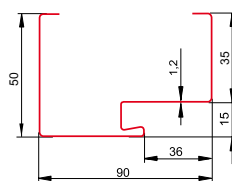
ościeżnica aluminiowa z przegrodą termiczną
