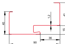
ościeżnica aluminiowa z przegrodą termiczną
